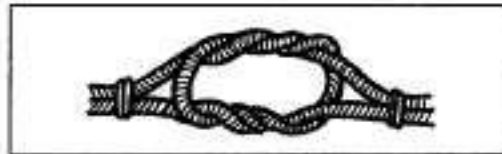
Двойной прямой. Соединение пеньковых и капроновых канатов при сильном натяжении.
