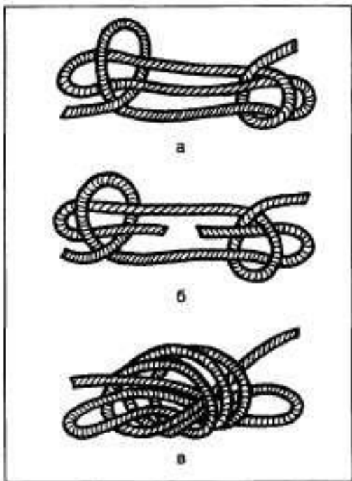
Укорачивающий: а — простой без обрыва; б-с обрывом; в — сложный. Укорачивание пеньковых и капроновых канатов без их разрезаний и с разрезанием.
