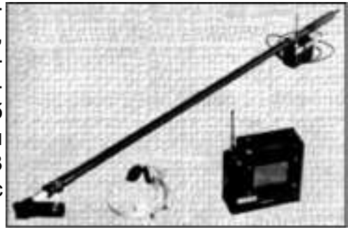
Прибор «Система-1К»
