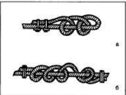
Штыковой: Соединение сталь-
