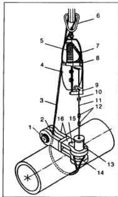
Автоматическое расстроповочное устройство ПАР-1: 1 — замок; 2 — ролик; 3 — строп; 4 — тывающая катушка; 5 — спир самонама- 6 — серьга; 7 — барабан; 8 — ось пружина; ; 9 — 10 — упор; 11 — канат управ узлолови-; 12 рабин; 13 — шпингалет; 14 — ш — ка-; 15 — жинный фиксатор; 16 — щеки
