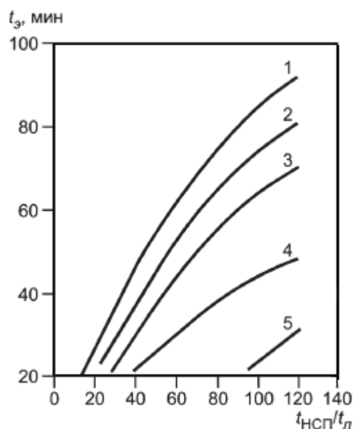
Рисунок P.3 - Зависимость эквивалентной продолжительности пожара t_3 от продолжительности пожара для железобетонных и огнезащищенных металлических конструкций перекрытия в условиях локальных пожаров t_{л} (или продолжительности НСП t_{НСП} ) при горении твердых и трудногорючих материалов
