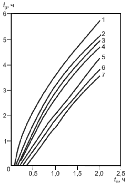
Рисунок Р.8 - Зависимость эквивалентной продолжительности пожара t_3 от характерной продолжительности объемного пожара t_{\text{П}} для железобетонных несущих стен
