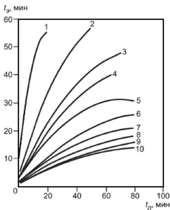
Рисунок Р.5 - Зависимость эквивалентной продолжительности пожара t_3 от продолжительности пожара t_{п} для горизонтальных незащищенных металлических конструкций
