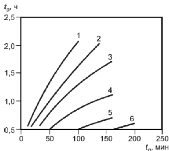
Рисунок Р.4 - Зависимость эквивалентной продолжительности пожара t_3 от продолжительности пожара t_{п} для железобетонных и огнезащищенных металлических конструкций перекрытия при горении ЛВЖ и ГЖ
