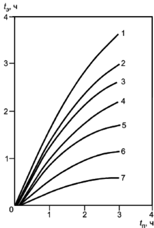
Рисунок Р.7 - Зависимость эквивалентной продолжительности пожара t_3 от характерной продолжительности пожара t_{П} для огнезащищенных металлических и железобетонных конструкций перекрытия
