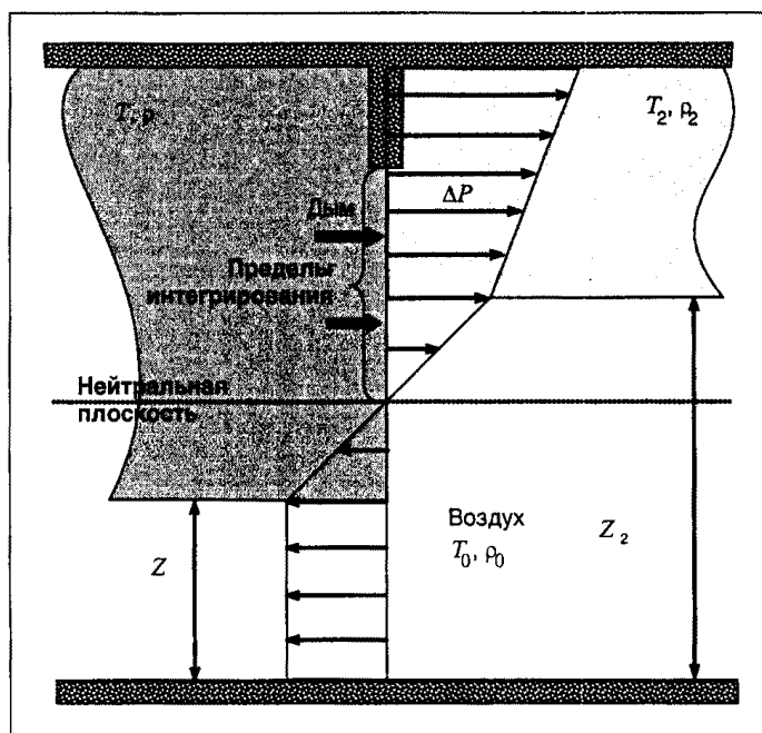
Рис. Пб.1. Массопотоки через проем
