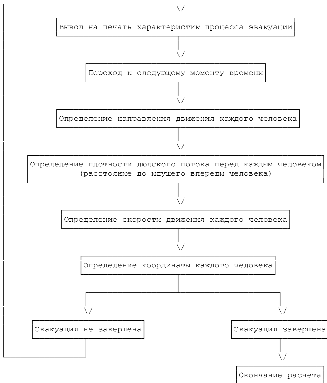
Рис. ПЗ.2. Блок-схема определения расчетного времени эвакуации людей из здания
